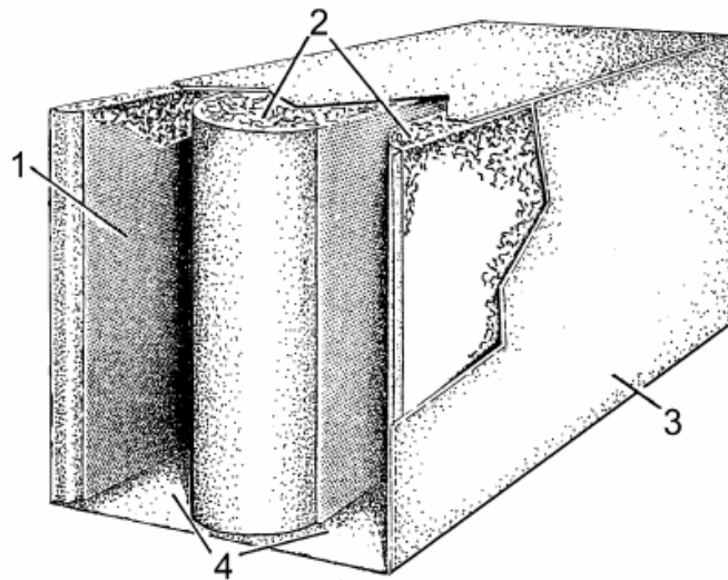
صدا خفه کن با صفحات مستطیلی موازی 1- ورق استیل مشبک گالوانیزه 2- فایبر گلاس باپشم های معدنی 3- جدار استیل 4- ورودیهای موثر در جذب
